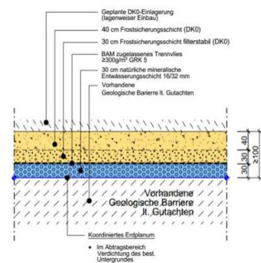
Abbildung 4 Regelaufbau Deponiebasis
